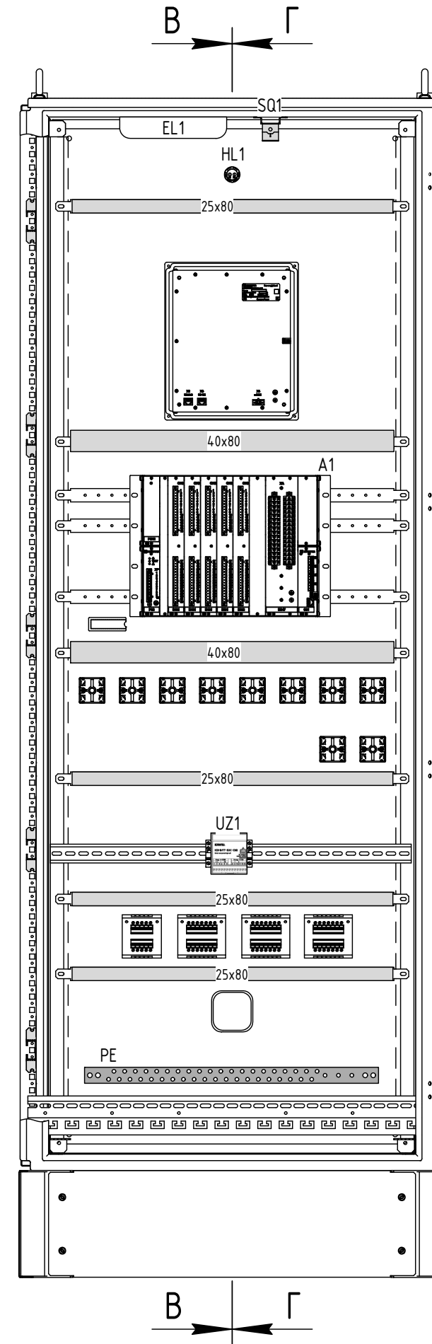
Вид сзади Дверь, ряды зажимов и вертикальные короба условно не показаны
